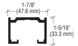
STANDARD D7 OVERHEAD TRACK SPECIFY D1027 ASSEMBLY
